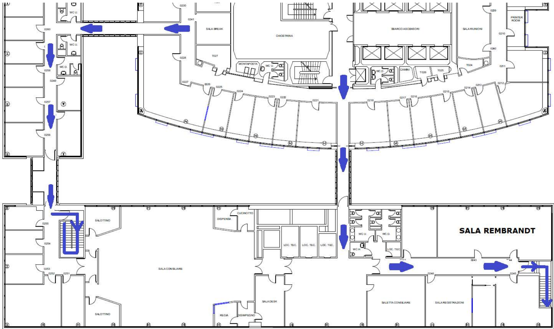
percorsi da seguire per accedere dal secondo piano al primo piano – corpo basso
