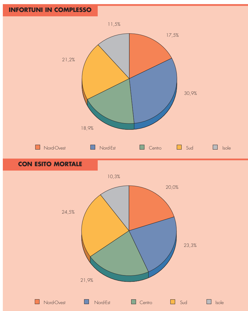
TAV. 3: DENUNCE DI INFORTUNIO IN AGRICOLTURA PER RIPARTIZIONE GEOGRAFICA - ANNO DI ACCADIMENTO 2017
