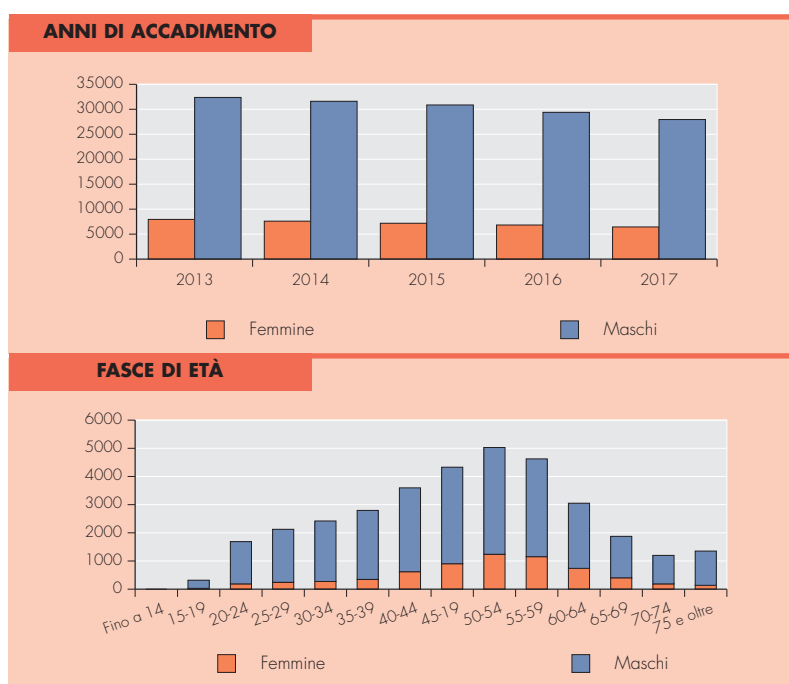
TAV. 1: DENUNCE DI INFORTUNIO NELLA GESTIONE AGRICOLTURA PER ANNO DI ACCADIMENTO, SESSO E FASCE DI ETÀ
