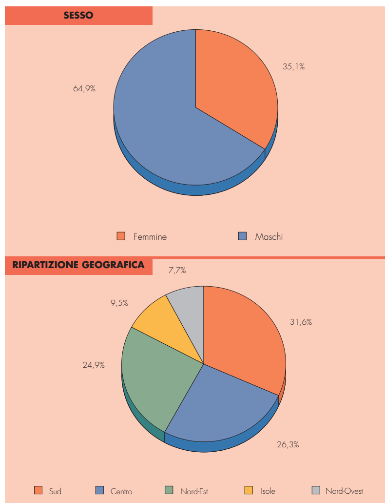
TAV. 3: MALATTIE PROFESSIONALI DENUNCIATE PER SESSO E RIPARTIZIONE GEOGRAFICA - ANNI DI PROTOCOLLO 2013 - 2017
