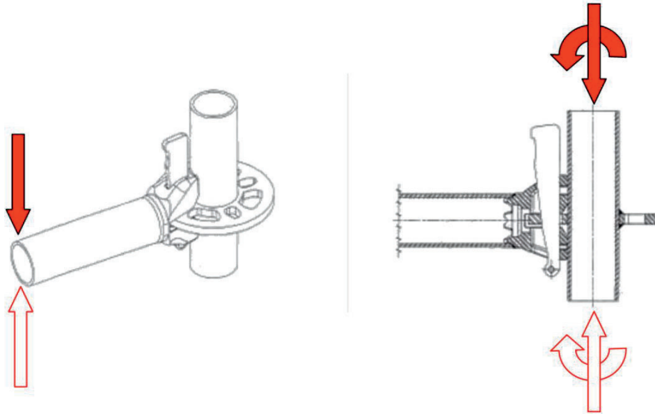
Figura 4.2.3-1 Schema di applicazione dello spostamento e azioni al nodo
