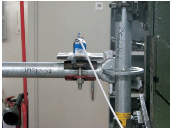
Figura 4.2.2.3-3: Inizio prova
