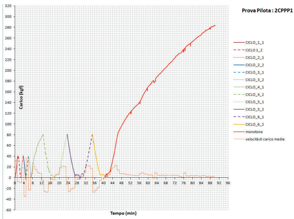
Figura 4.2.4-2 Curva carico-tempo. Velocità di carico media (kg f /min).
