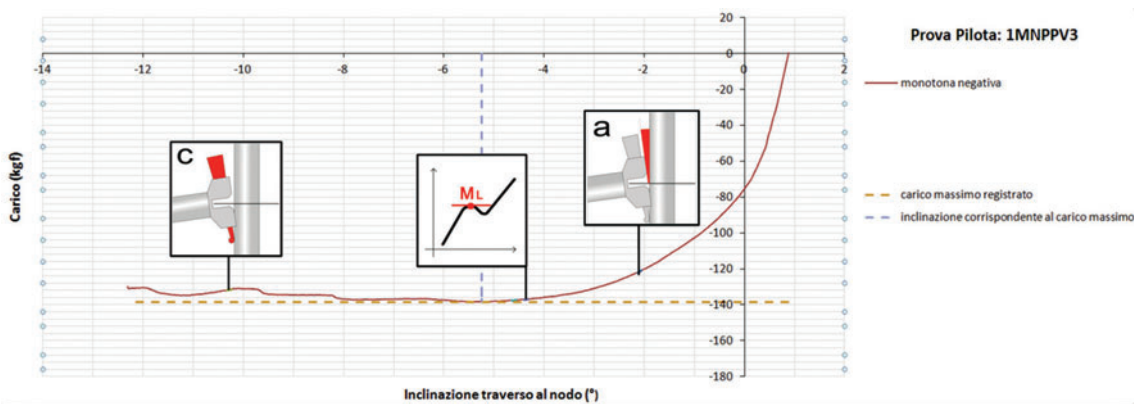
Figura 4.2.1.3-2: Curva carico-inclinazione del traverso al nodo. Carico massimo registrato e inclinazione corrispondente. Individuazione dei punti A e C corrispondenti al verificarsi degli eventi a e c descritti in figura 4.1-3. Individuazione del punto M_L corrispondente ad un massimo locale della curva.
