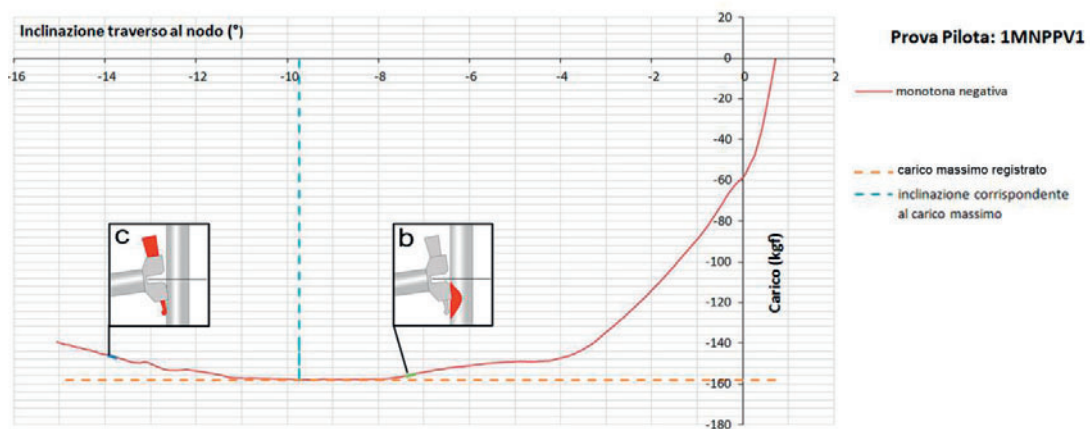
Figura 4.2.2.1-2: Curva carico-inclinazione del traverso al nodo Carico massimo registrato e inclinazione corrispondente. Individuazione dei punti B e C corrispondenti al verificarsi degli eventi b e c descritti in figura 4.1-3
