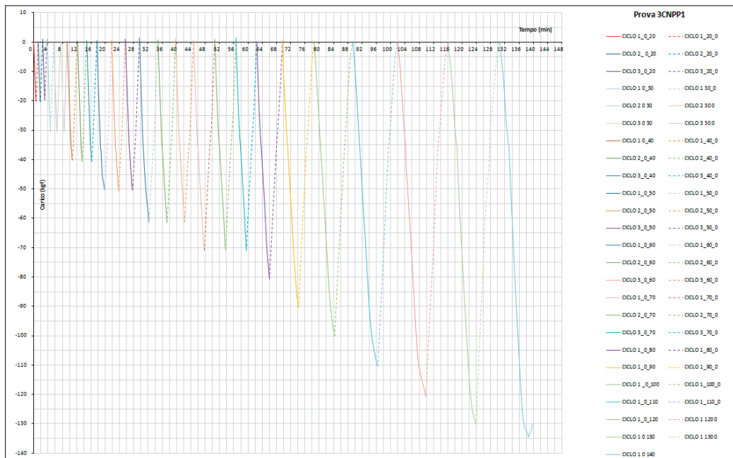
Figura 4.2.5-1 Curva carico-tempo. Velocità di carico media (kg f /min).
