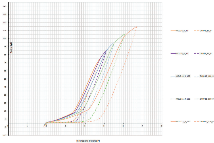
Figura 4.2.8-5 Curva parziale carico-inclinazione trasverso al nodo
