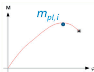
Figura 3.2.1-1. Schematizzazione di una prova pilota del tipo monotona nel verso positivo dello spostamento (I metodo) per la valutazione di R_k^+
