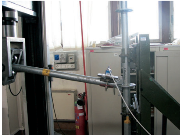
Figura 4.2.2.4-6: Fine prova
