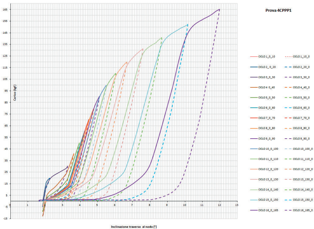
Figura 4.2.8-2 Curva carico-inclinazione traverso al nodo
