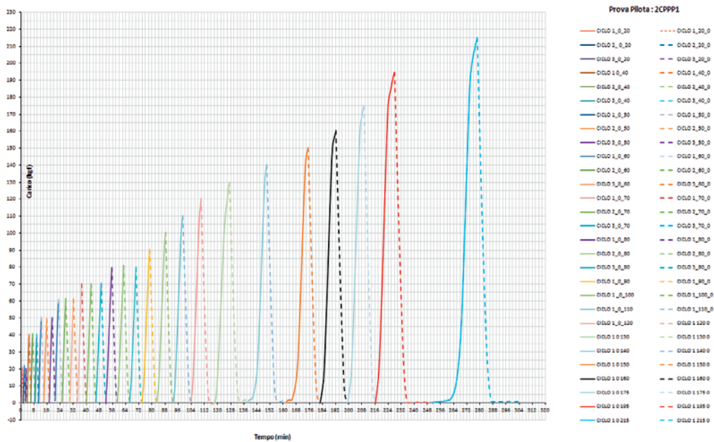
Figura 4.2.6-2: Curva carico-tempo
