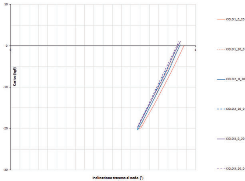
Figura 4.2.5-3 Curva parziale carico-inclinazione traverso al nodo
