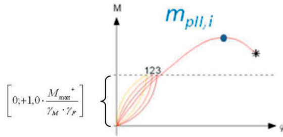
Figura 3.2.2-1. Schematizzazione di una prova pilota del tipo ciclica senza inversione di carico (II metodo) per la valutazione di R_k
