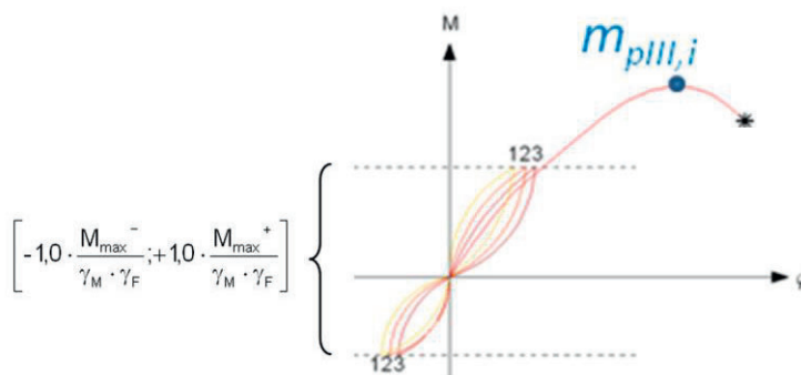
Figura 3.2.3-1. Schematizzazione di una prova pilota del tipo ciclica senza inversione di carico (III metodo) per la valutazione di R_k
