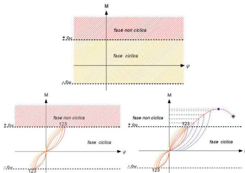
Figura 1-1 Schematizzazione della prova a collasso per la valutazione della resistenza del dispositivo di collegamento con rottura nel verso positivo del carico in accordo al punto 7.2 della UNI EN 12811-3:2005.
