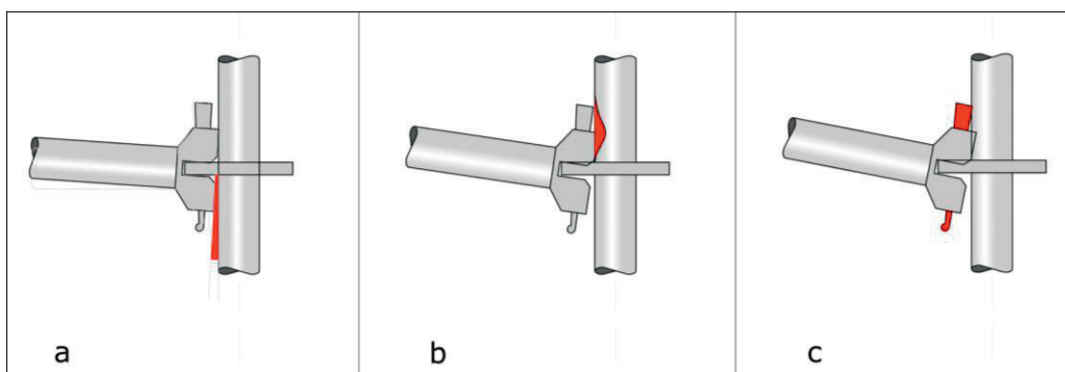
Figura 4.1-4 Schematizzazione degli eventi macroscopici rilevati ad occhio durante le prove con spostamento imposto positivo: a. formazione di aria al contatto tra montante e forchetta del traverso; b. imbozzamento del montante al contatto con il traverso; c. contatto fra cuneo e montante.
